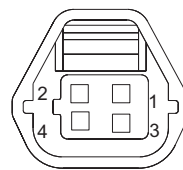
C_RPA sensor_RL MID 后左中倒车雷达传感器
