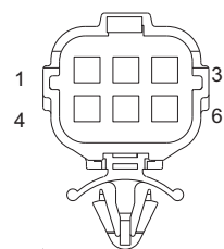
C_Camera_REAR 倒车影像后摄像头
