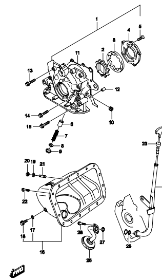
1230 МАСЛЯНЫЙ НАСОС И ПОДДОН
