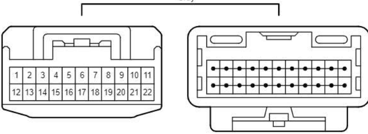
90980-12372
