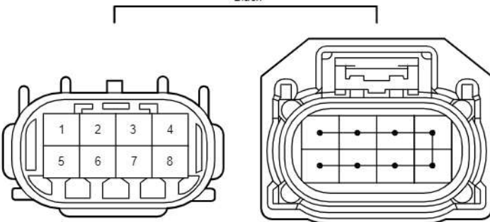
90980-12B56
