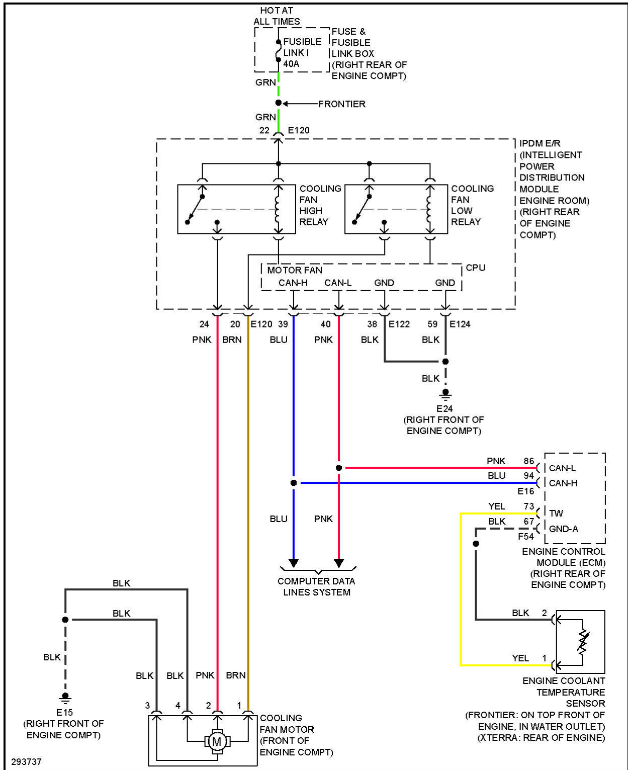
Fig. 12: 4.0L, Cooling Fan Circuit
