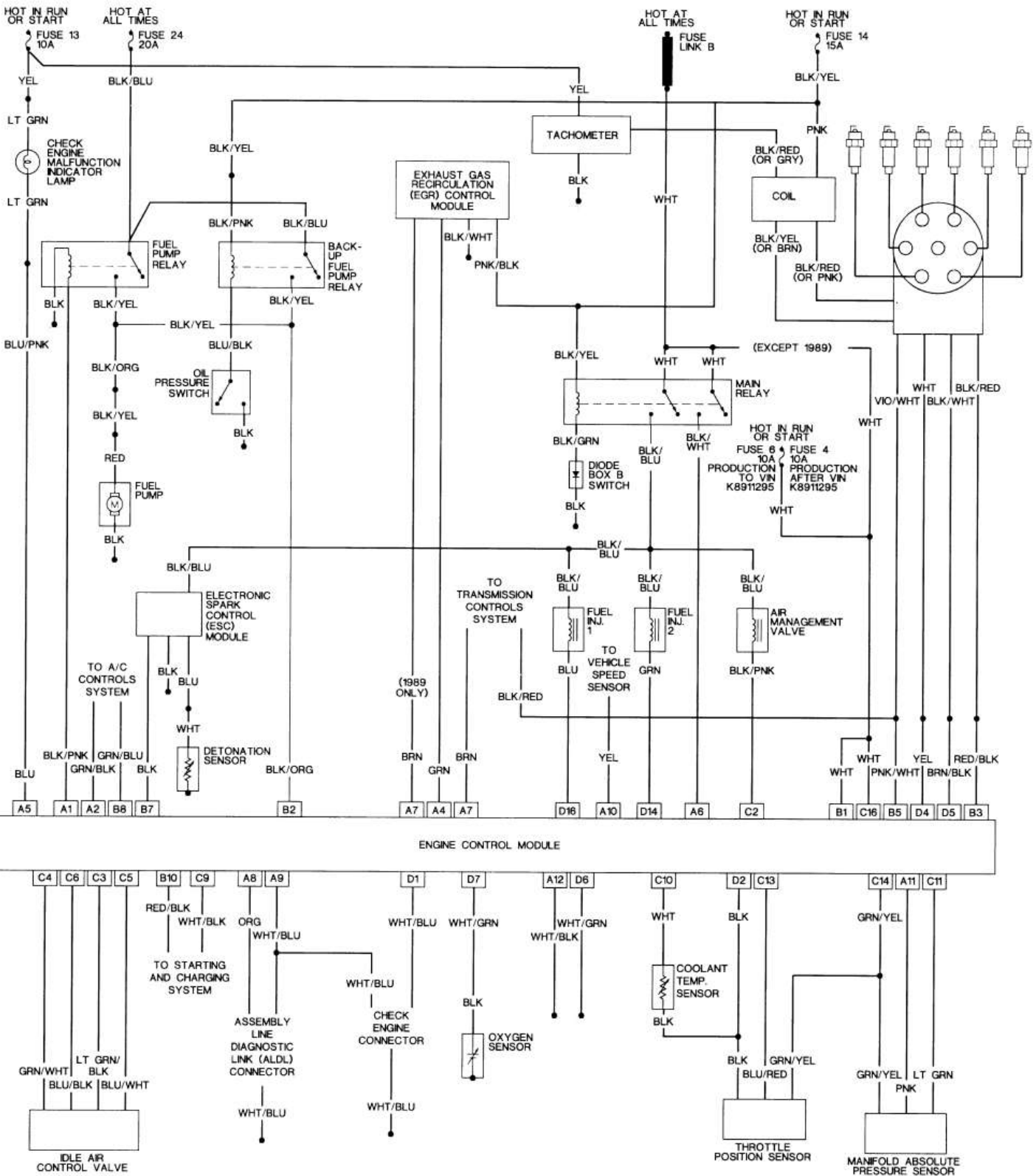
Higo. Higo. 59: Motor cableado de control Trooper diagrama de 1989-1991 II con el motor 2.8L
