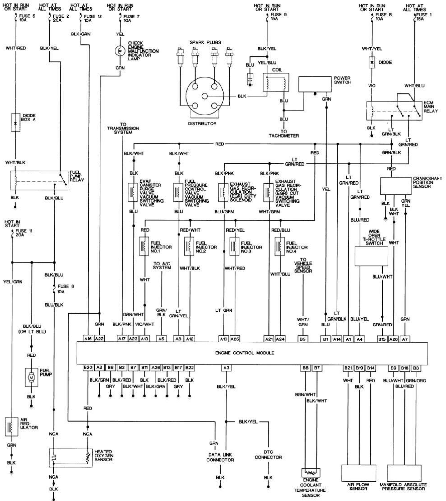
Higo. Higo. 46: Motor diagrama de cableado de control 1995 pick-up con el motor 2.6L
