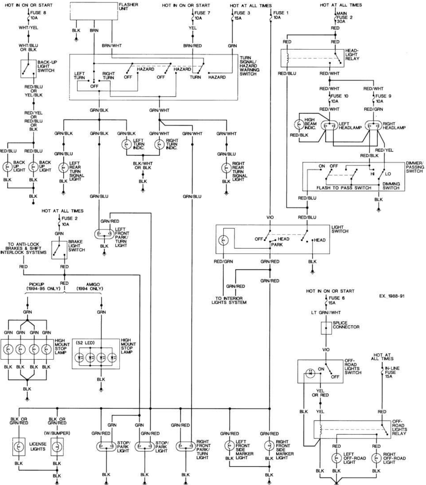
Higo. Higo. 44: diagrama de cableado del chasis (continuación) -1998-95 Amigo y Pick-up
