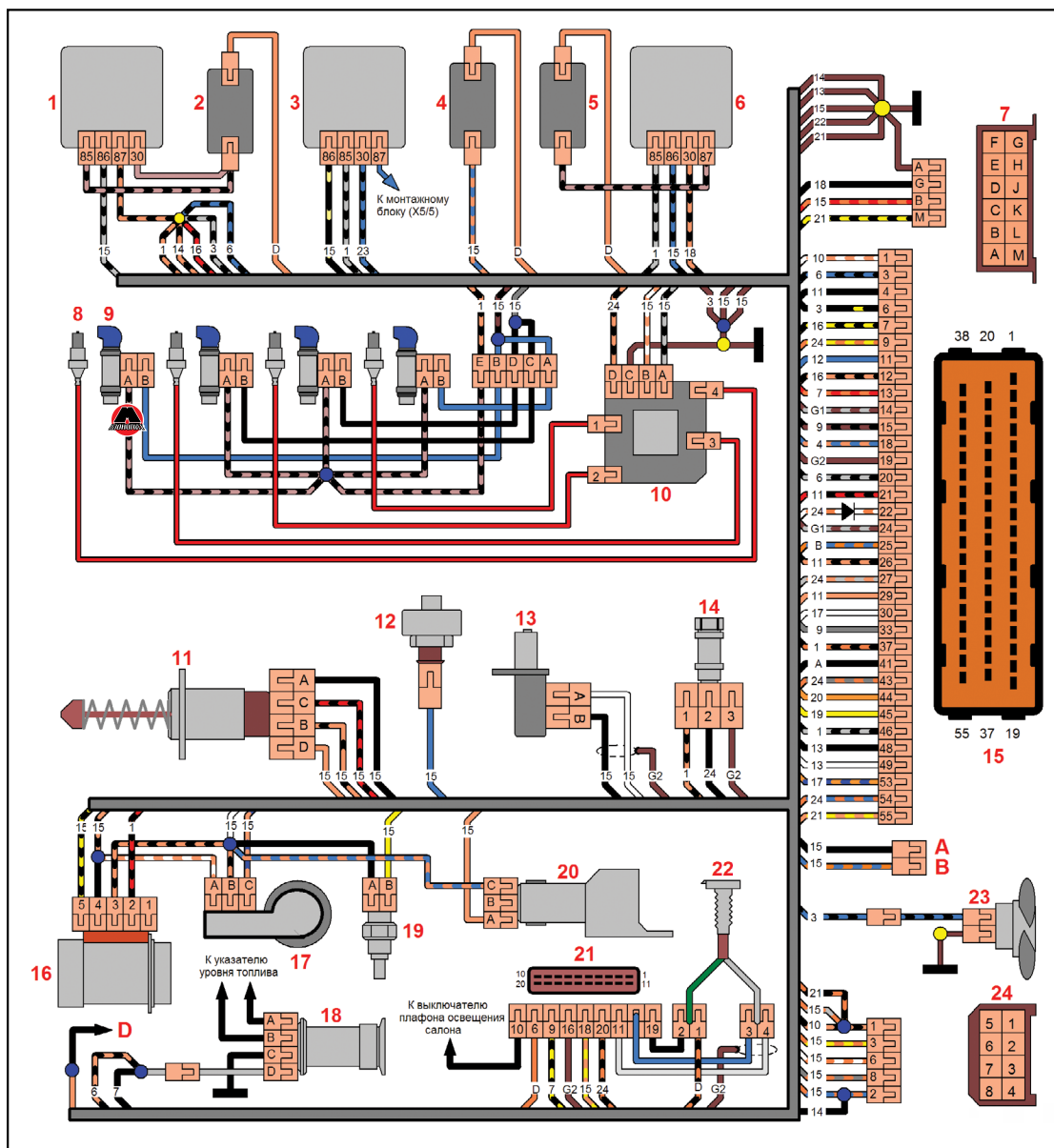
СХЕМА СОЕДИНЕНИЙ СИСТЕМЫ УПРАВЛЕНИЯ ДВИГАТЕЛЕМ ВАЗ-2111 С РАСПРЕДЕЛЕННЫМ ВПРЫСКОМ ТОПЛИВА ПОД НОРМЫ ТОКСИЧНОСТИ СТРАН СНГ (КОНТРОЛЛЕР M1.5.4) АВТОМОБИЛЕЙ ВАЗ-21083, ВАЗ-21093, ВАЗ-21099:
