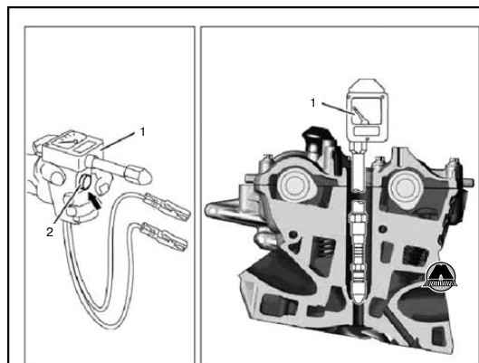
1. Компрессометр. 2. Контактный выключатель.
