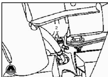
Сливная пробка радиатора системы охлаждения
